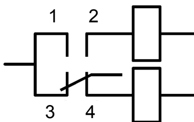
Рисунок А4 Схема электрическая принципиальная выключателей
