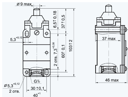
Рисунок А1 Выключатель ВП15К21А211
