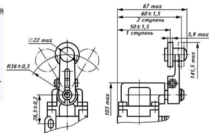
Рисунок А3 Выключатель ВП15К21А231 (остальное см. рис. А1)
